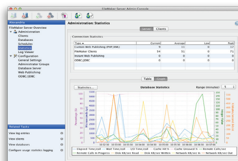
Das Statistik-Diagramm der Admin-Konsole zeigt Ihnen in Echtzeit verschiedene Datenbankauswertungen.
